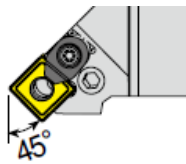
PSSNR/L (Lever Type 45°)
