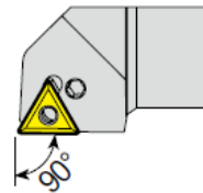
PTGNR/L (Lever Type 90°)
