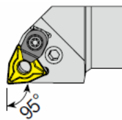
PWLNR/L (Lever Type 95°)
